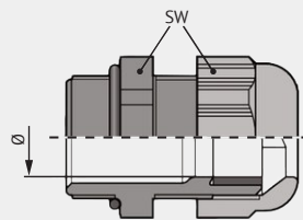
Schnitt Kabelverschraubung
