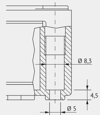
Schnitt durch Montagelöcher
